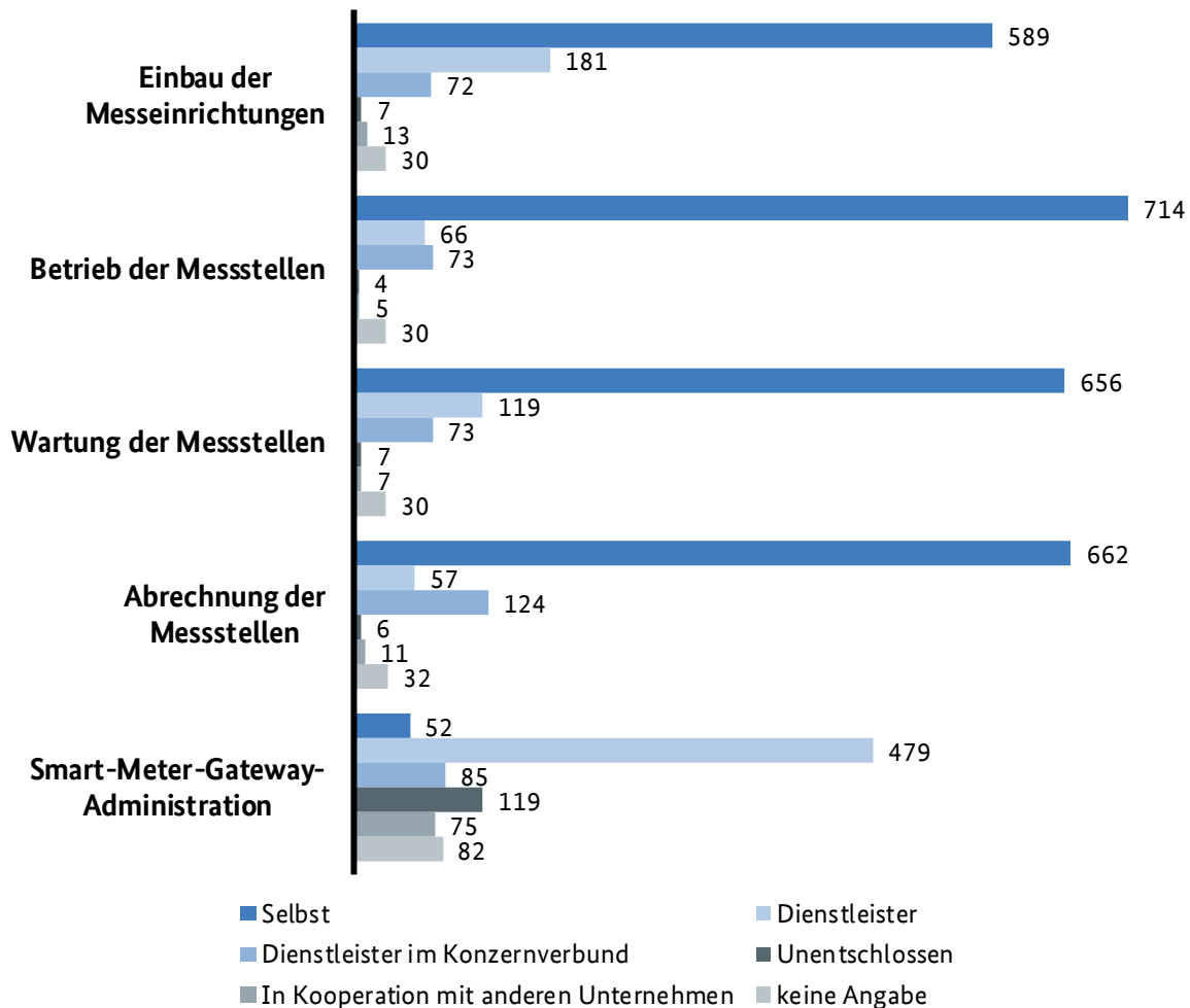
Abbildung 140: Art der Ausführung der Funktionen des Messstellenbetriebs
