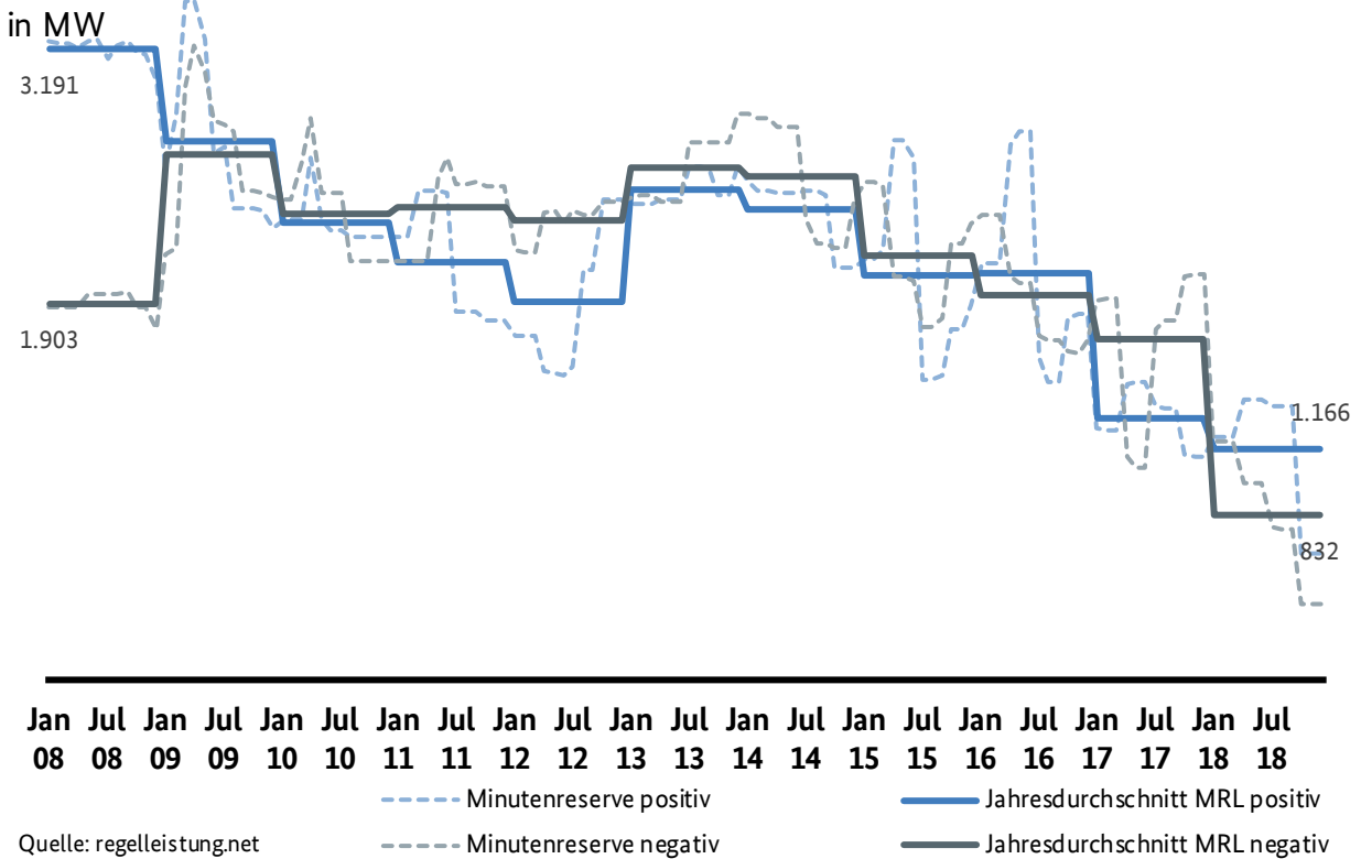
Abbildung 82: Entwicklung der insgesamt ausgeschriebenen Minutenreserveleistung in den Regelzonen von 50Hertz, Amprion, TenneT und TransnetBW
