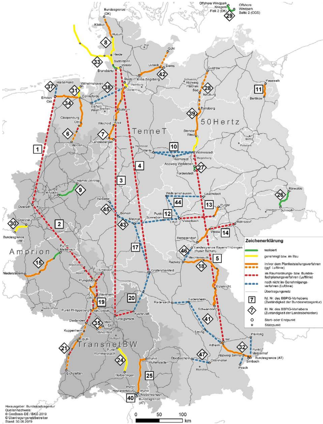
Abbildung 37: Stand der Ausbautvorhaben nach dem Bundesbedarfsplangesetz (BBPIG); Stand: 2. Quartal 2019
