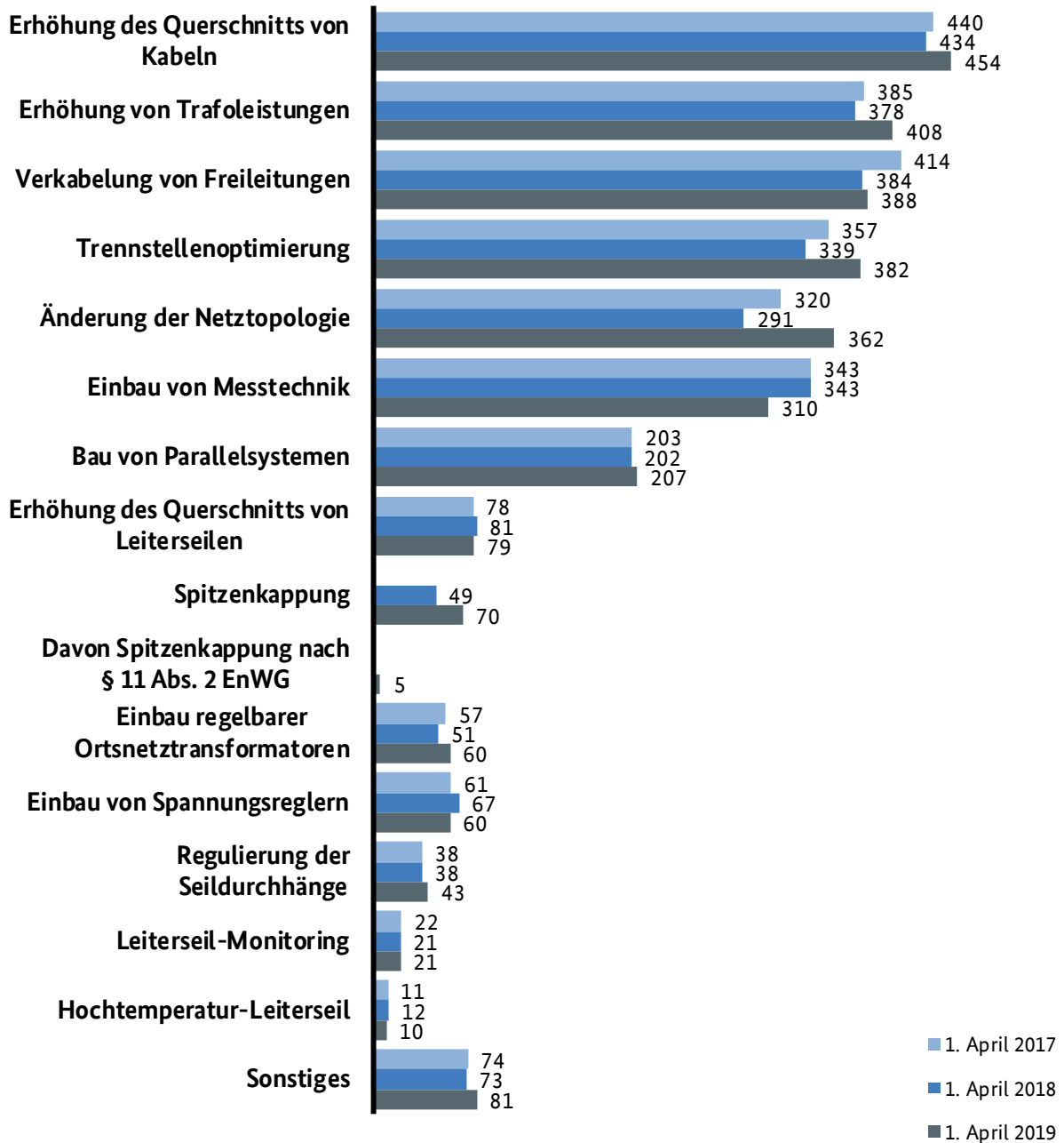
Abbildung 40: Überblick angewandeter Maßnahmen zur Netzoptimierung
