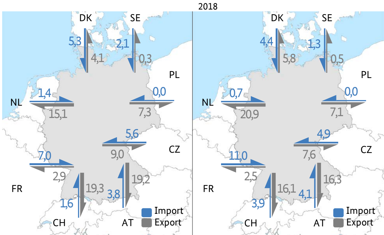
Abbildung 97: Physikalische Lastflüsse
