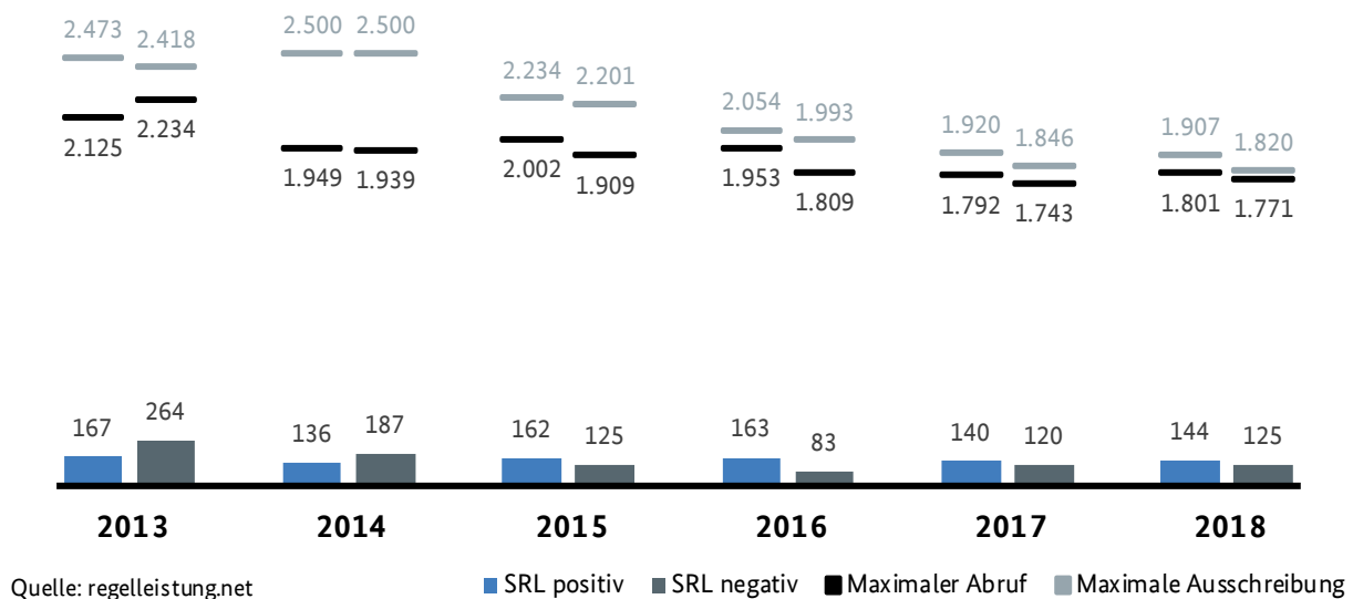
Abbildung 83: Durchschnittlicher Einsatz von Sekundärregelleistung inkl. Bezüge und Lieferungen im Rahmen der Online-Saldierung beim NRV
