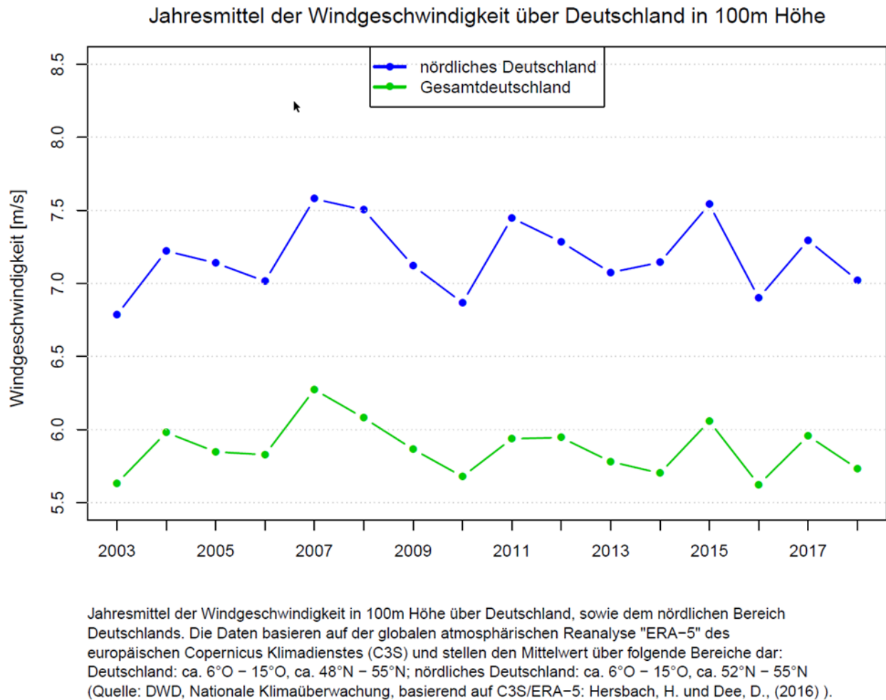
Abbildung 27: Jahresmittel der Windgeschwindigkeit in 100 m Höhe über Deutschland, sowie dem nördlichen Bereich Deutschlands
