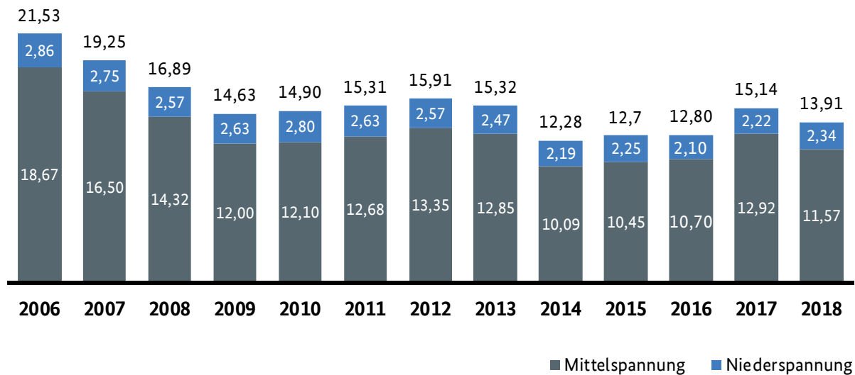
Abbildung 51: Entwicklung des SAIDI EnWG in der NS und MS von 2006 bis 2018
