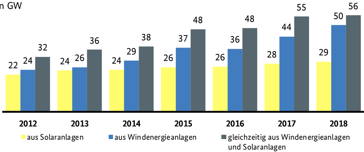
Abbildung 28: Maximale Einspeisung
