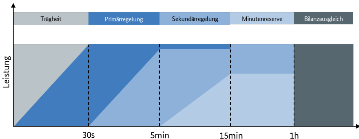
Abbildung 79: Schematische Darstellung des Einsatzes der Regelreservearten im zeitlichen Ablauf
