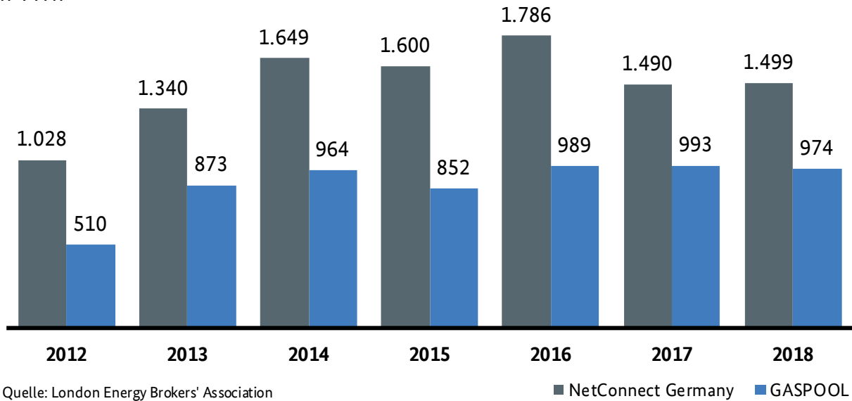
Abbildung 198: Entwicklung der Erdgashandelsvolumina der in der LEBA organisierten Brokerplattformen für deutsche Marktgebiete
