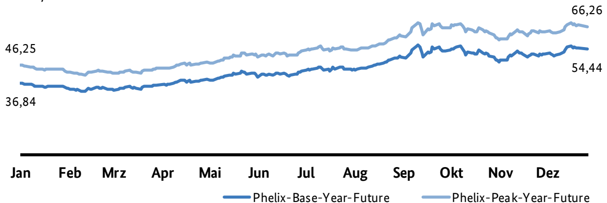
Abbildung 110: Preisentwicklung der Phelix-DE-Frontjahres-Futures im Jahresverlauf 2018
