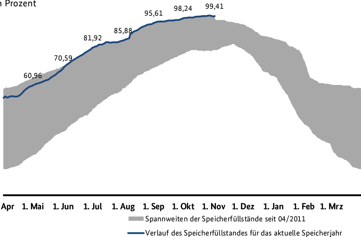
Abbildung 164: Verlauf der Gasspeicherfüllstände in Deutschland – Stand: 1. November 2019
